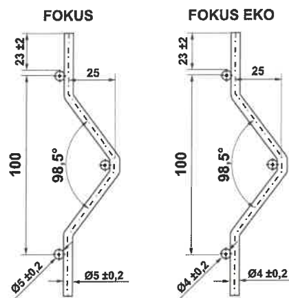
Wszystkie wymiary w mm
